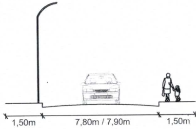
PERFIL TRANSVERSAL SEM ESCALA
