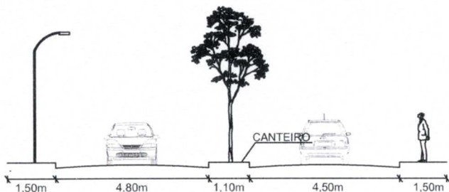
PERFIL TRANSVERSAL
