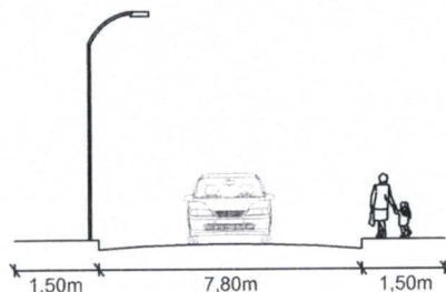
PERFIL TRANSVERSAL SEM ESCALA
